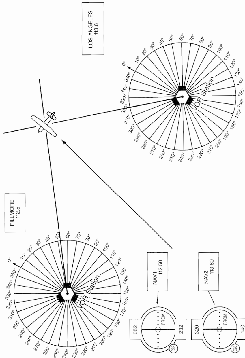
Figure 18. VOR Crosschecking
