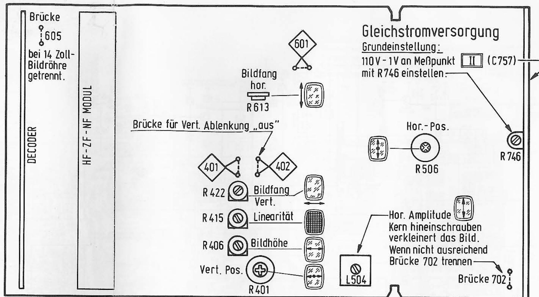
Einsteller und Testpunkte auf der Chassisplatte, Bestückungsseite.
