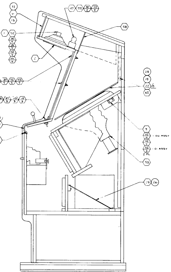
SECTION A-A
