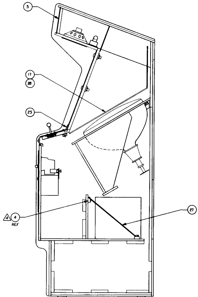
SECTION A-A
