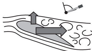
Hebel vollständig zurückgezogen Flügel überzogen Schwacher Auftrieb – Hoher Luftwiderstand Starkes Rütteln
