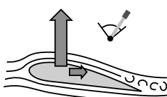
Manche tiré vers l'arrière Angle d'attaque fort Portance élevée – traînée modérée Légère turbulence
