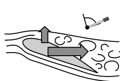
Manche tiré vers l'arrière Aile décrochée Portance faible – traînée importante Turbulence élevée
