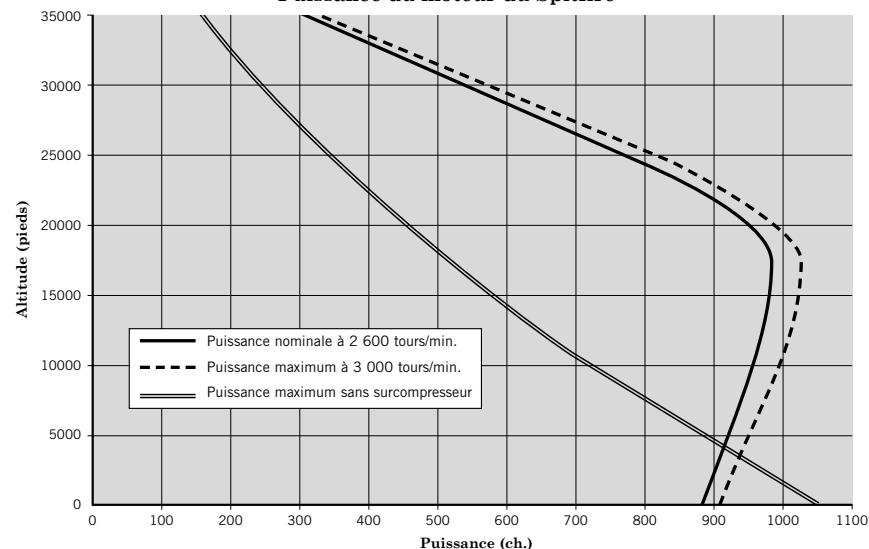
Puissance du moteur du Spitfire
