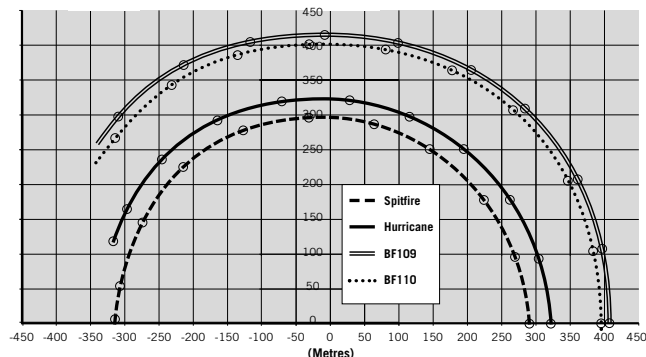
Performances en virage à 16 000 pieds
