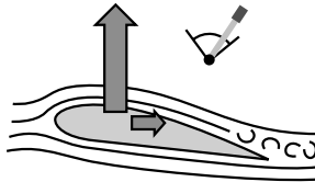
Barra indietro Alto angolo di incidenza Alta portanza – media resistenza Lieve scuotimento
