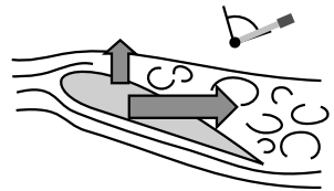
Barra tutta indietro Ala in stallo Bassa portanza – alta resistenza Forte scuotimento
