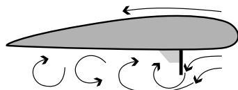
Aerofreno di picchiata aperto (alta resistenza)
