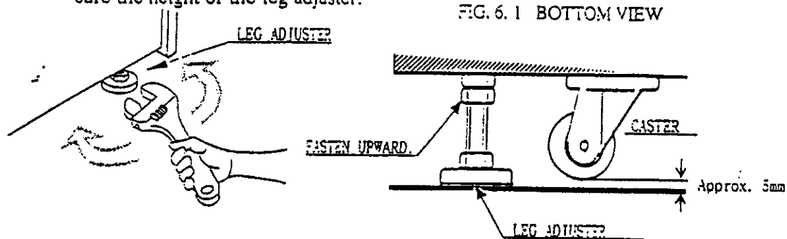
FIG. 6. 2 LEG ADJUSTER
